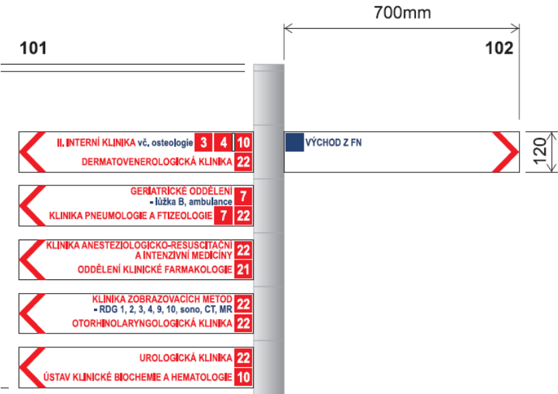
ROZVINUTÝ POHLED 101 - 102
