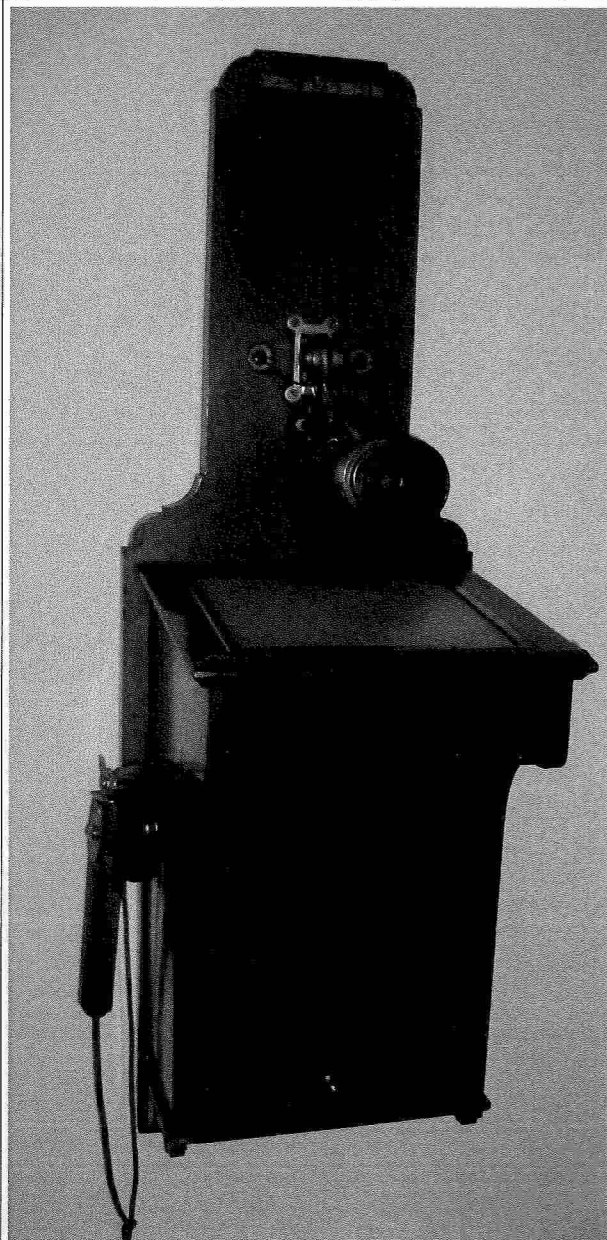
8. 22702 Nástěnný pultový telefonní přístroj MB
