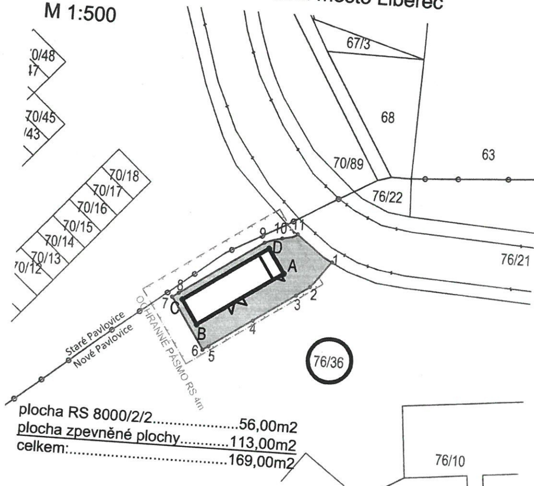
vytyčovací souřadnice RS 8000/2/2
