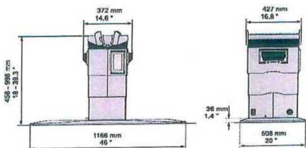
Mobilní sloupek, verze C
