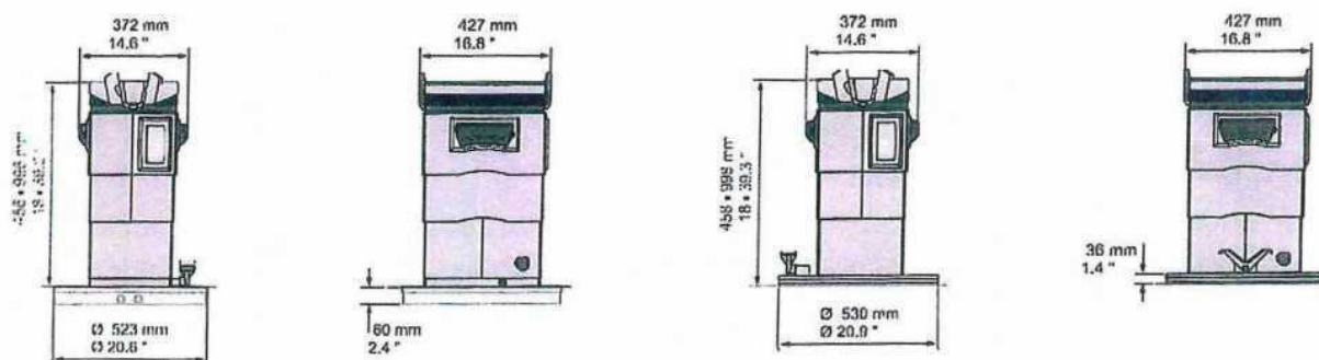
Stabilní sloupek, verze B
