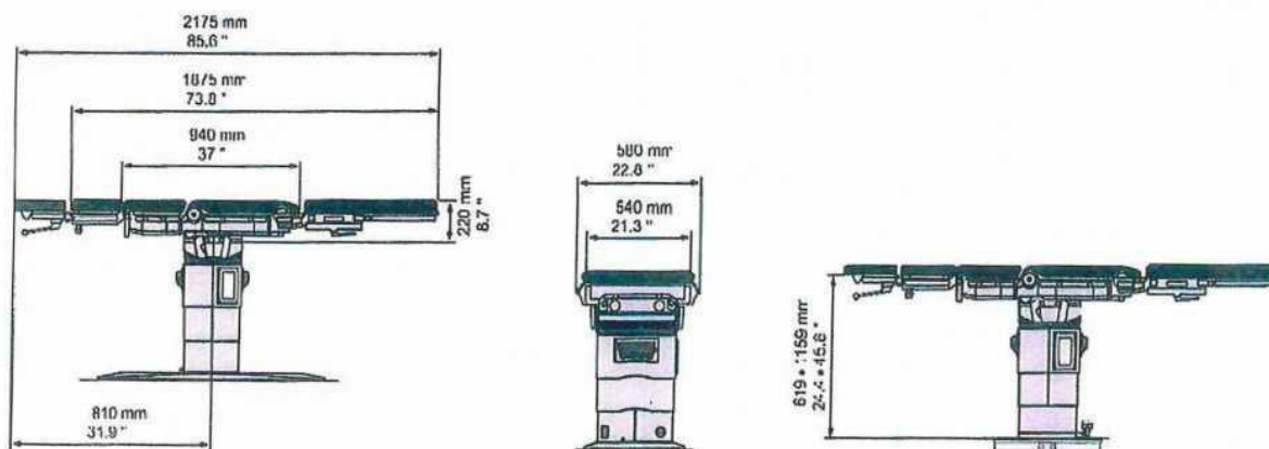
Rozměry desky stolu a rozsah výšek
