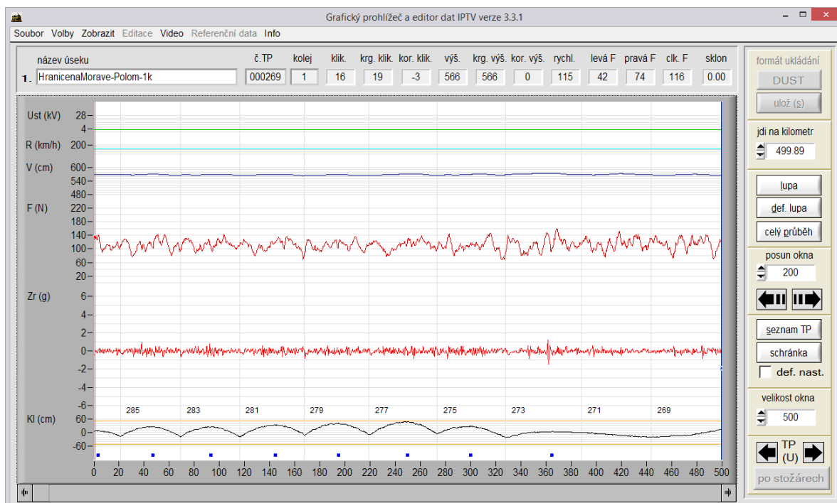
Obrázek 4 příklad zobrazení měřených dat IPTV systému
