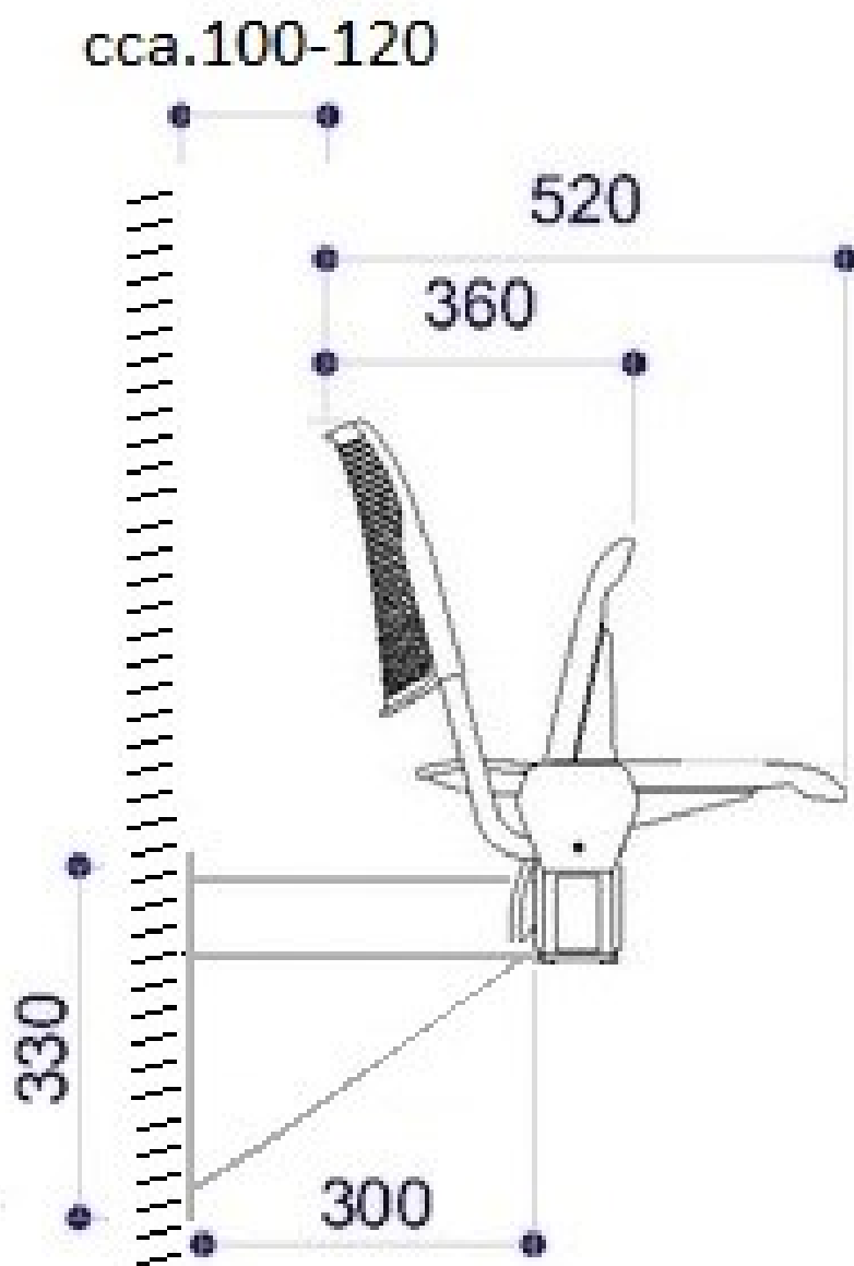
Schématický řez konzole a uchycení sedákového segmentu.
