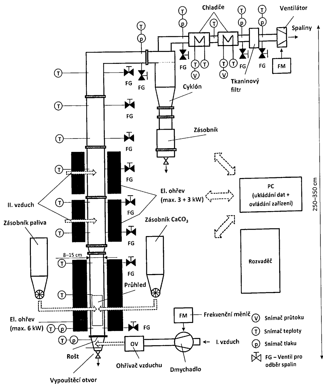
Obr. 1: Schéma prototypového výzkumného standu pro studium energetického využití pevného produktu torefakce
