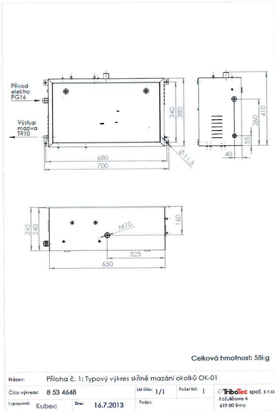
obr. č.1. Typový výkres skříňe mazání okolků OK-01
