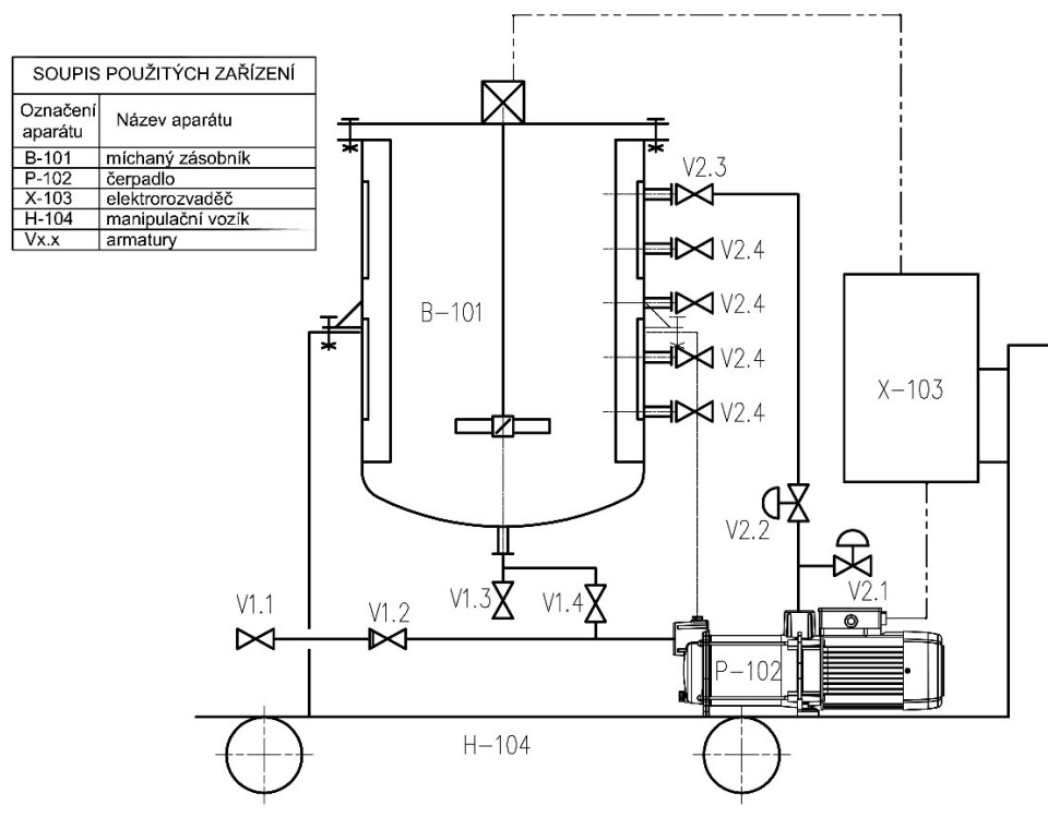
Obr. 1. Sestava míchané nádrže
