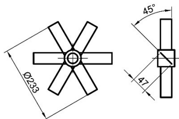
DETAIL GEOMETRIE MÍCHADLA
