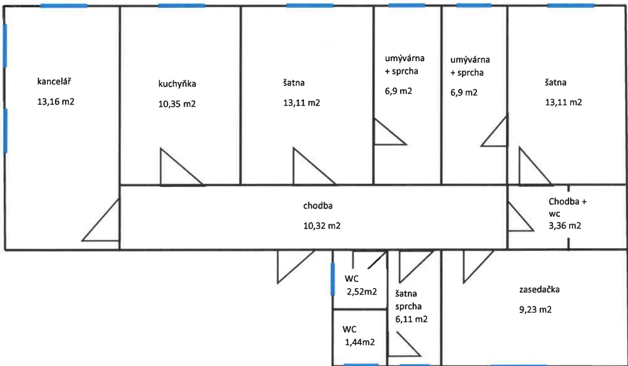
Areál skládky Suchý důl, administrativní objekt (půdorys bez měřítka)
