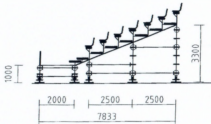
Řez tribunou - VIP část
