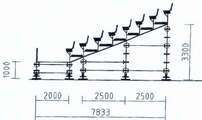
Řez tribunou - levá a pravá část
