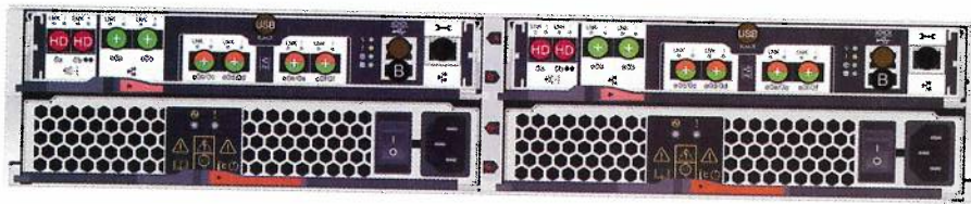
Obrázek: Konektivita diskového pole FAS2750
