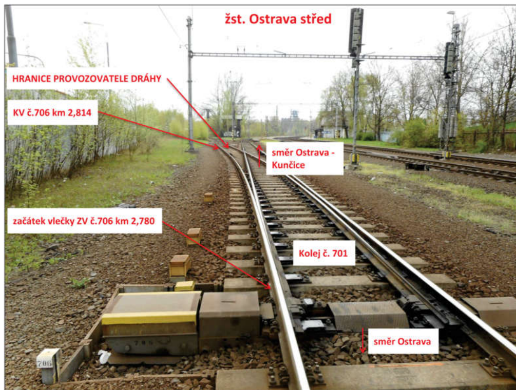
Obrázek č. 6: fotografie výhybky č. 706
