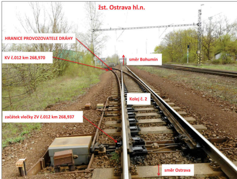
Obrázek č. 4: fotografie výhybky č. 012
