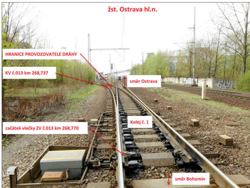
Obrázek č. 5: fotografie výhybky č. 013
