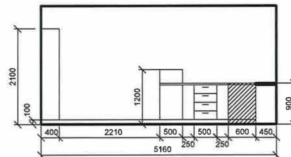
POHLED - B
