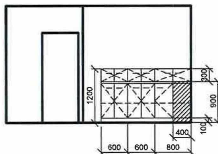
POHLED - D
