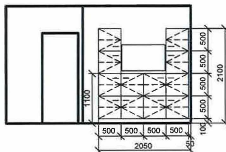
POHLED - E
