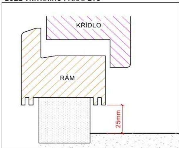
VÝŠKA ČISTÉ PODLAHY U AL PRAHU
