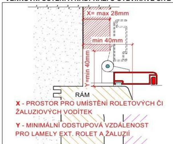
VENKOVNÍ OSTĚNÍ A NADPRAŽÍ U OTEVÍRÁVÉ SÍTĚ
