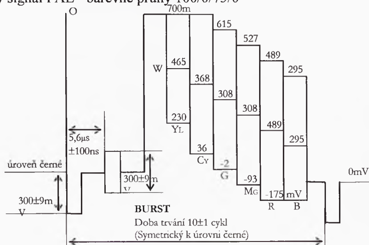
Úplný signál PAL - barevné pruhy 100/0/75/0
