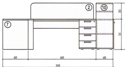
POHLED PŘEDNÍ
