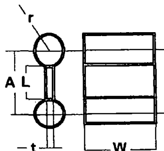
Obr. 1: Schéma zkušebního tělesa kde: r=3\text{mm} , L=4\text{ mm} , A= 10\text{mm} , W=100\text{mm} , t=0,5\text{mm}
