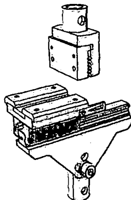
Obr. 1: Upínací čelisti
