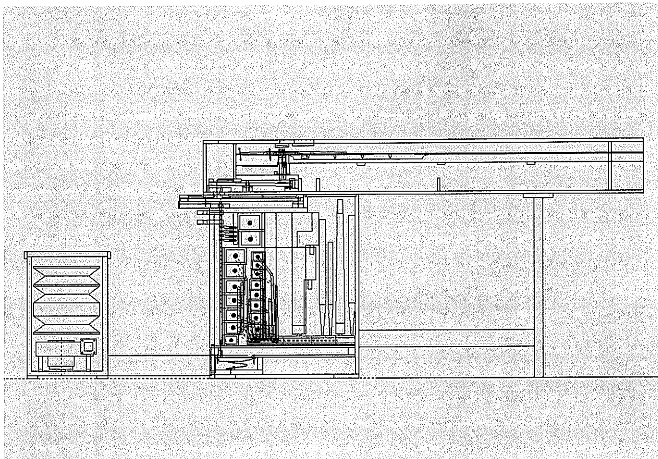
Schéma spojení cembala a pozitivu jak bylo vyrobeno do Jihlavy
