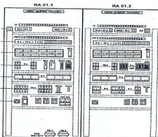
Měření a regulace Rozvaděč RA 01
