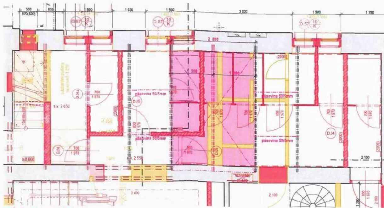
půdorys 1NP
