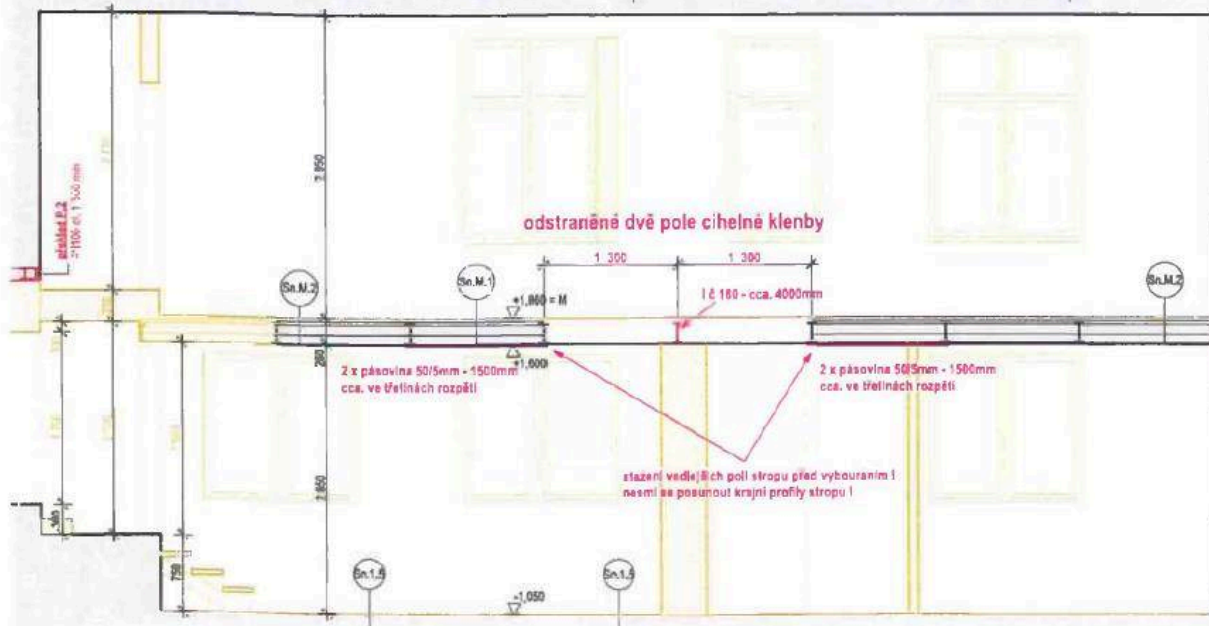
řez - bourání
