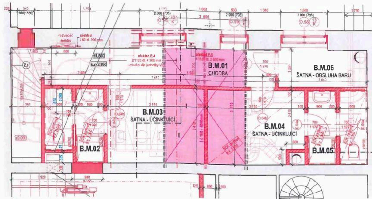
půdorys mezipatra
