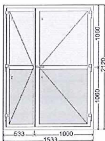
dveře vnitřní pohled (interiér)
