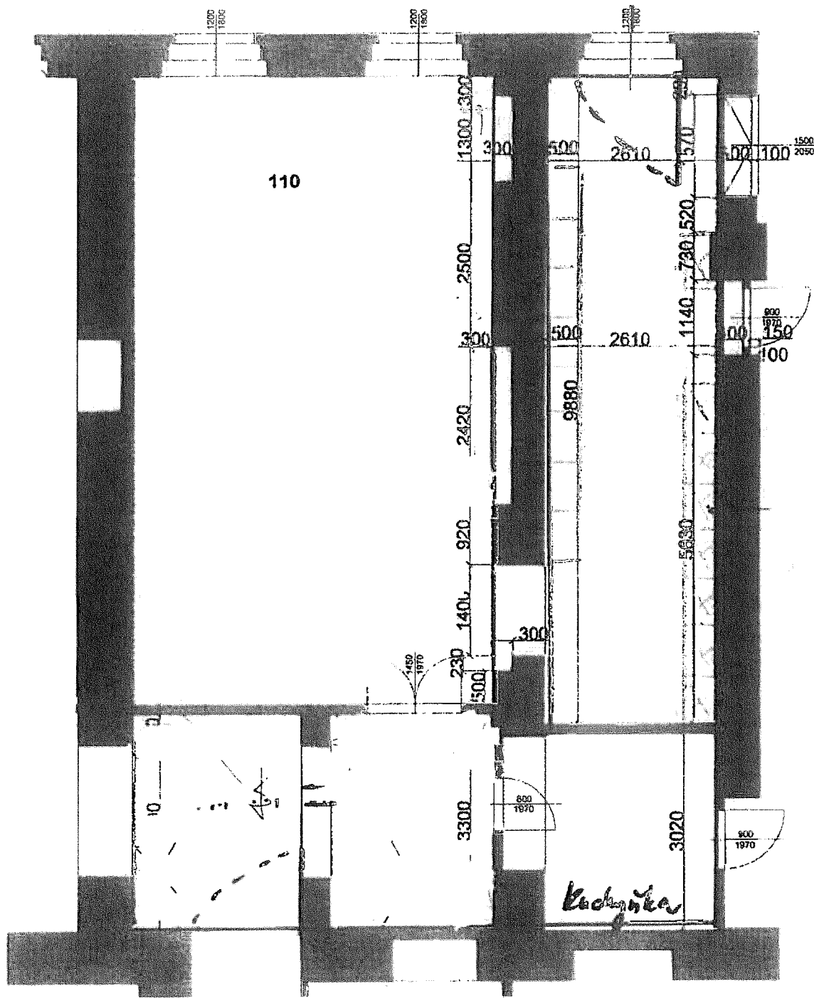
Národní dům na Vinohradech Praha 2, nám. Míru 9 Mezanin- služby 110 M-1:50
