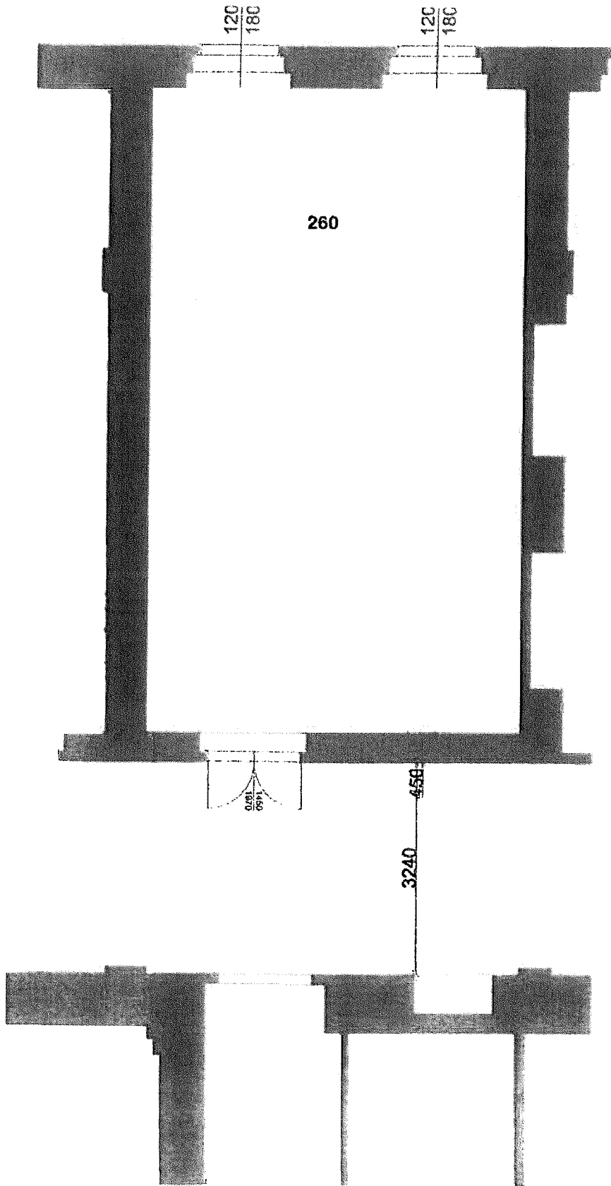
Národní dům na Vinohradech Praha 2, nám. Míru 9 1.Patro-kanceláře č.260 M-1:50
