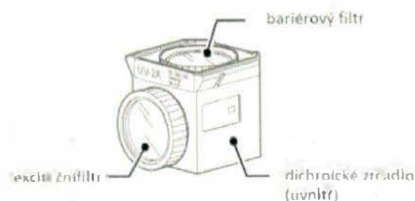
kostka s fluorescenčními filtry
