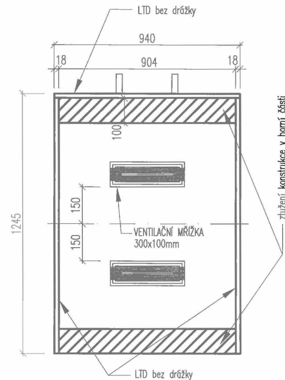
PŮDORYS
