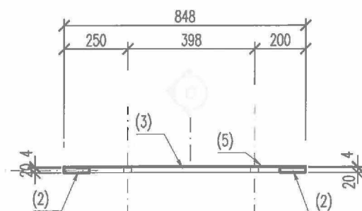
ŘEZ B
