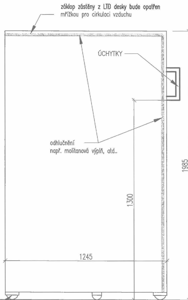
BOČNÍ POHLED
