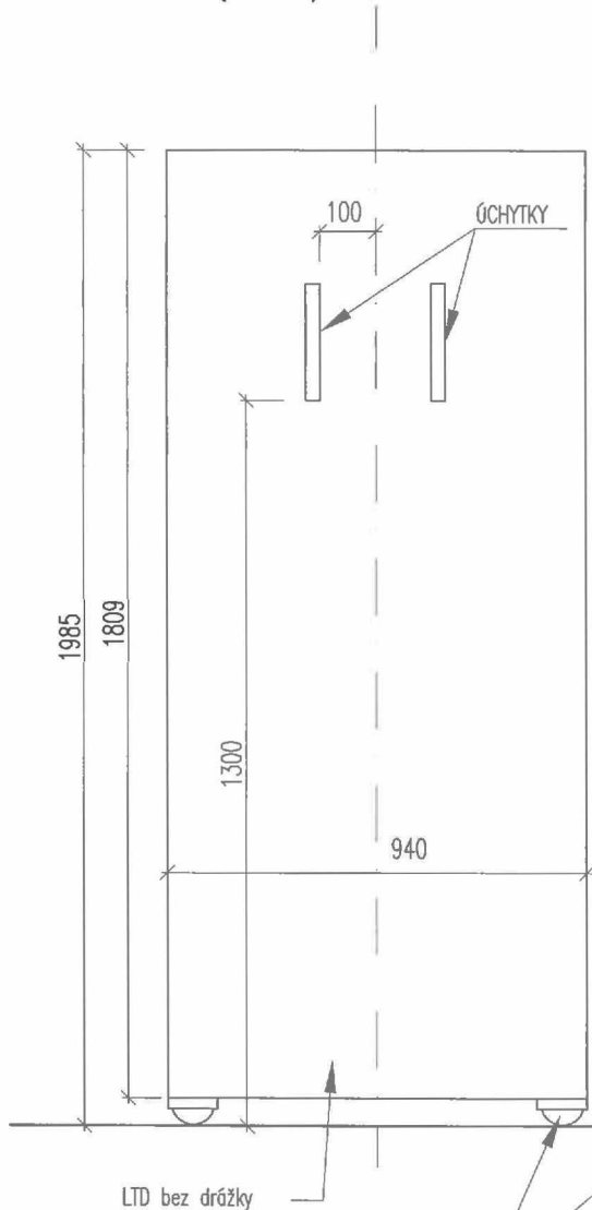
ČELNÍ (ZADNÍ) POHLED
