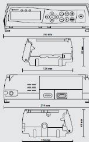
8713050 Infusomat® Space
