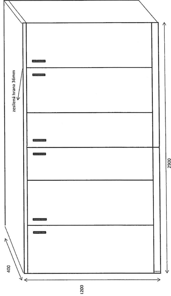
kancelář II. sestava na pravo Materiál: LTD H 1582 ST15
