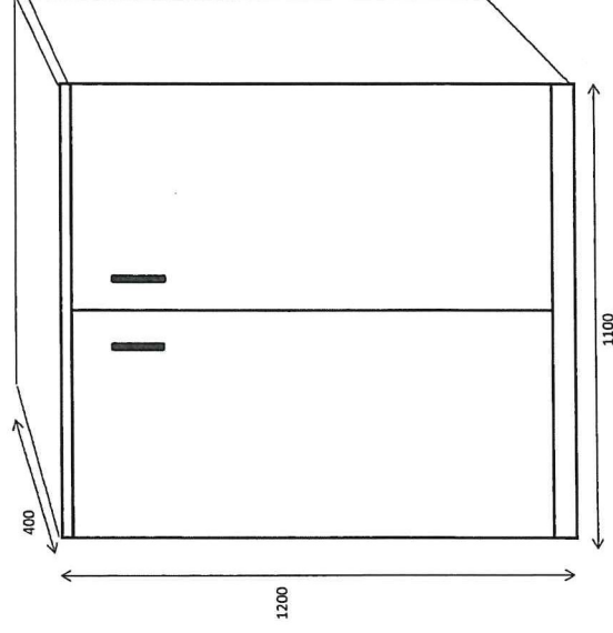
kancelář II. - skříňka u okna Materiál: LTD H 1582 ST15
