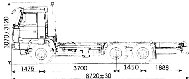
Výškové rozměry platí pro zatížené vozidlo
