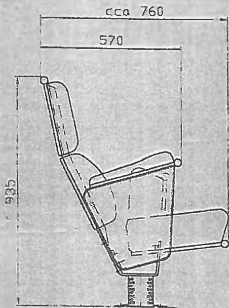
KŘESLO KRAJOVÉ
