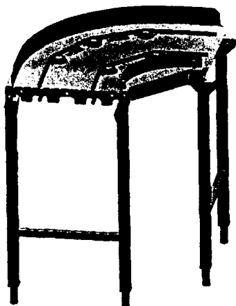
Manipulační stoly k tunelovým košovým myčkám
