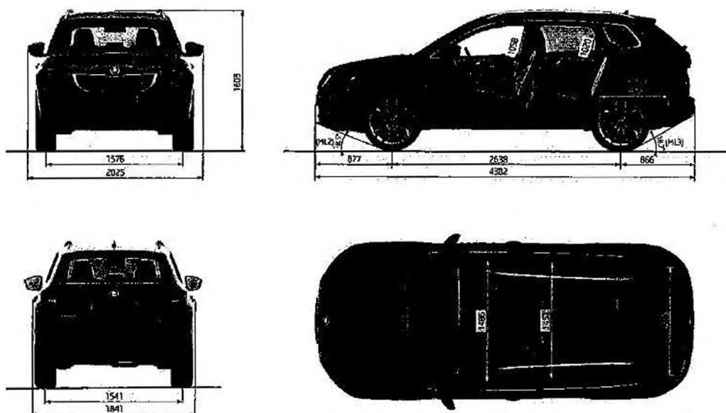
Rozměry nabízeného vozu
