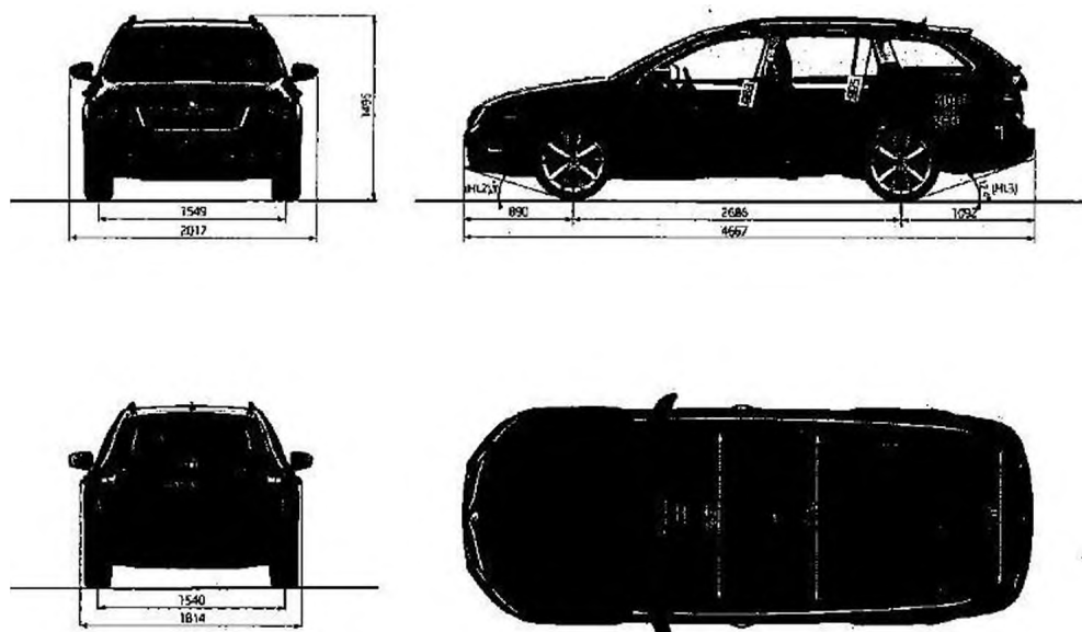
Rozměry nabízeného vozu
