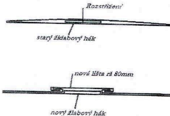
Schéma klempířské úpravy u žlabových háků
