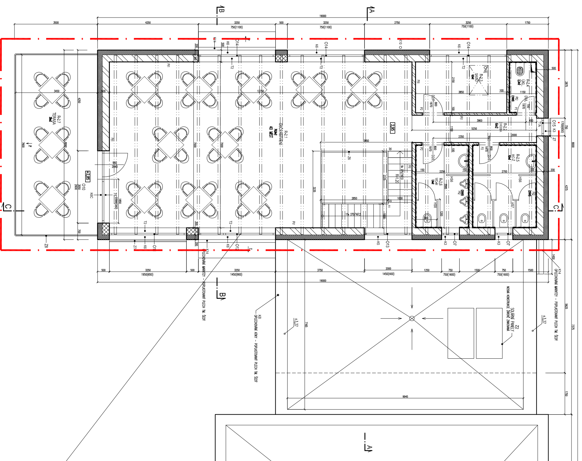
RESTAURACE 2.NP - VYMEZENÍ PLOCHY A MÍSTNOSTÍ
