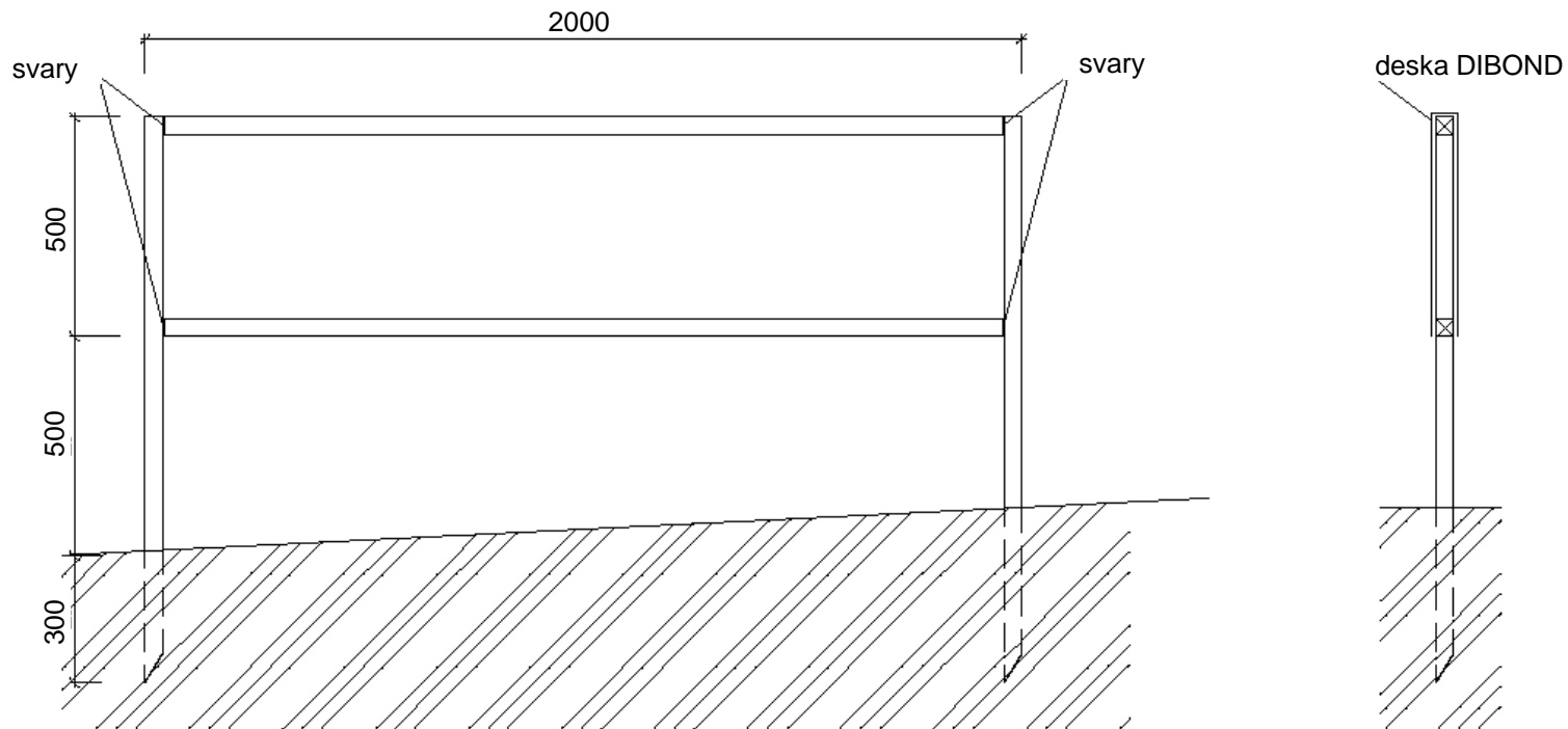
POHLED NA KONSTRUKCI RÁMU 1:10
