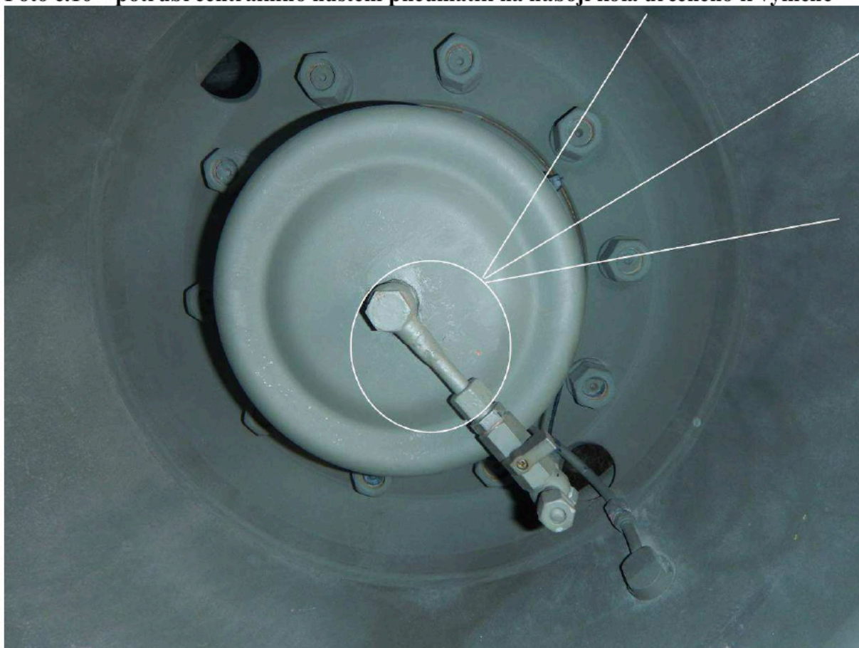
Foto č.10 – potrubí centrálního huštění pneumatik na náboji kola určeného k výměně
