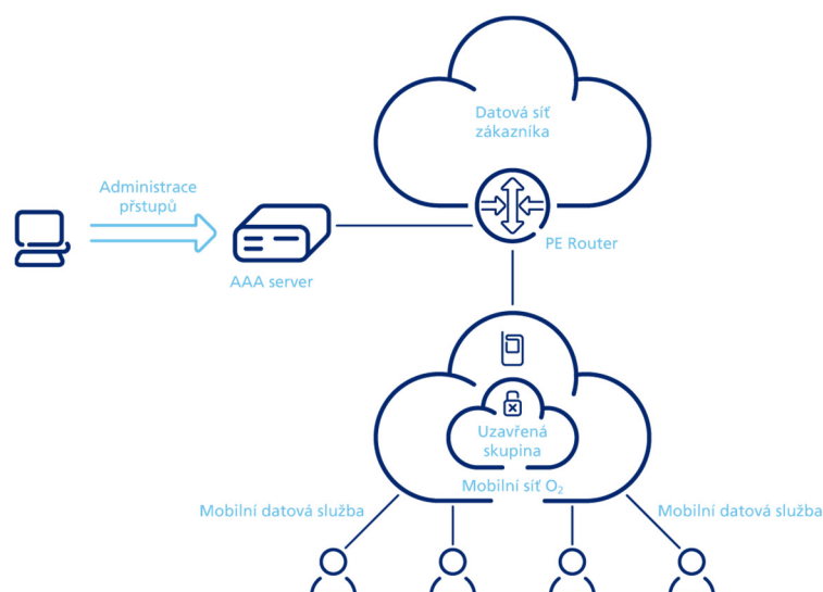
Obrázek 6 – Schéma služby IP Connect CMA s využitím přístupové služby O2 Remote Access
