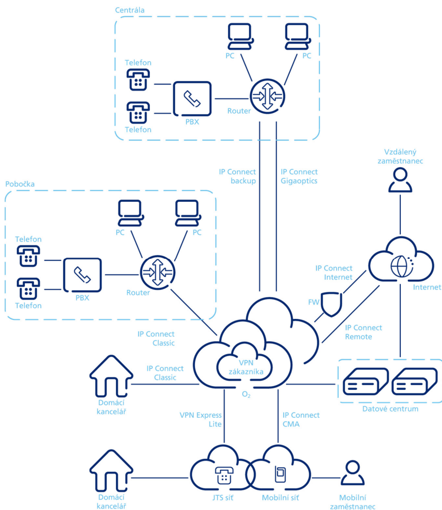
Obrázek 7 – Ilustrační příklad topologie služby IP Connect
