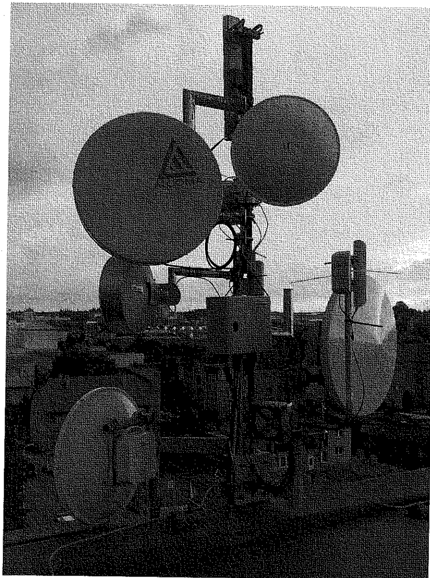
Foto 1 Rozmístění antén
