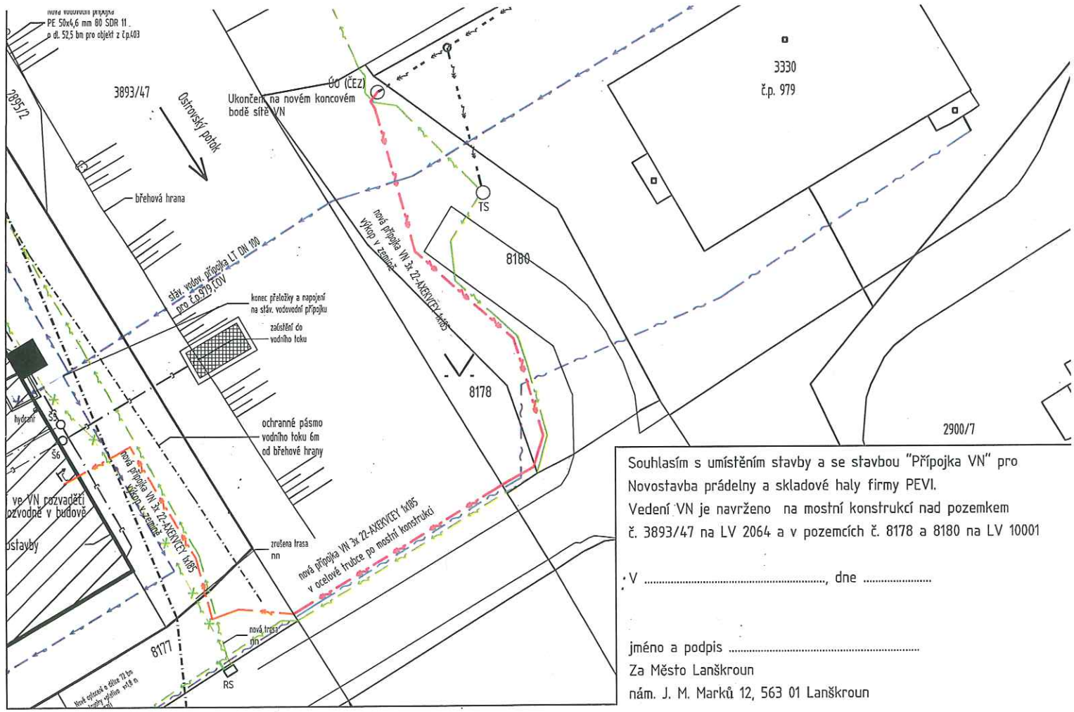
Situace vedení přípojky VN 1:250
