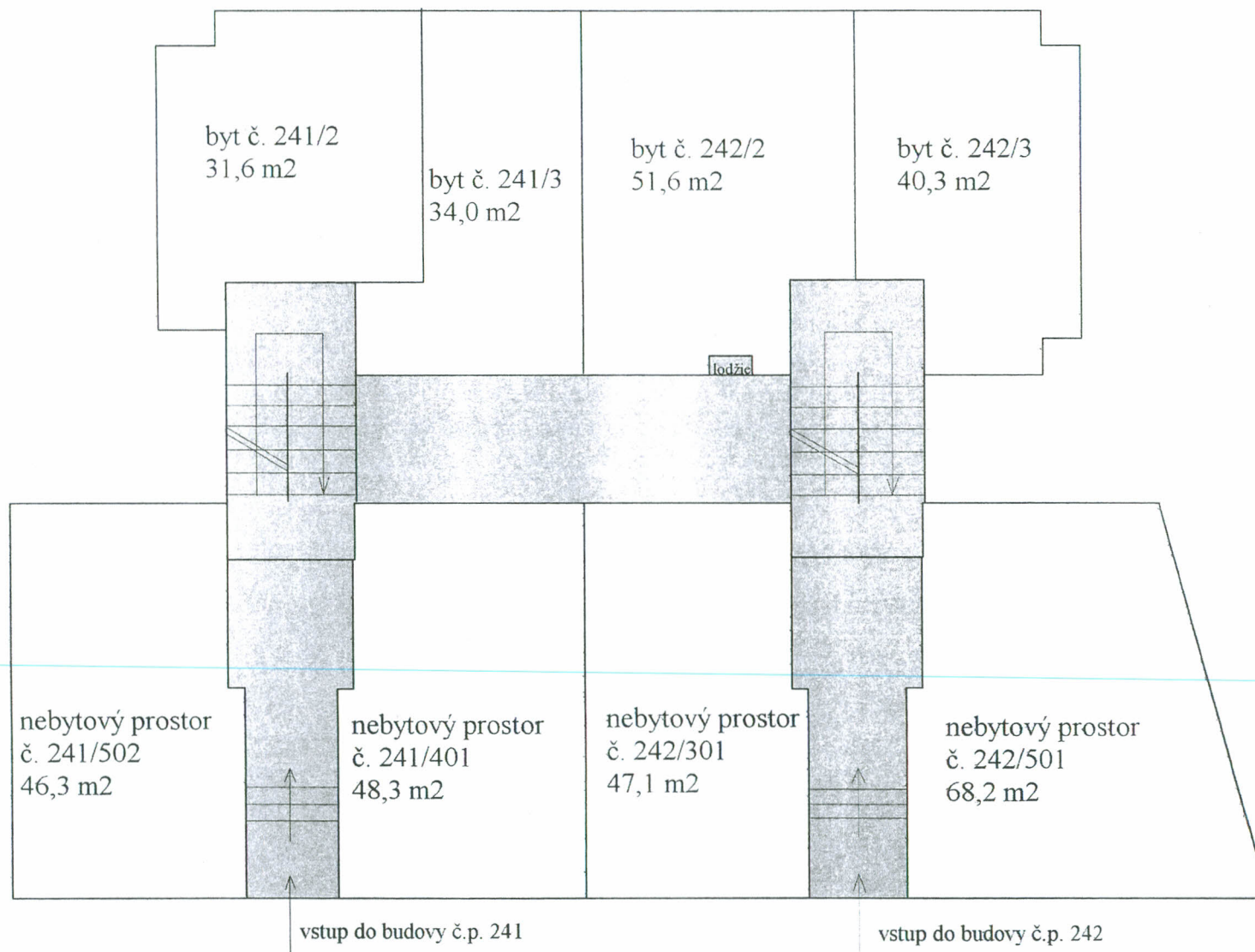
1. nadzemní podlaží
