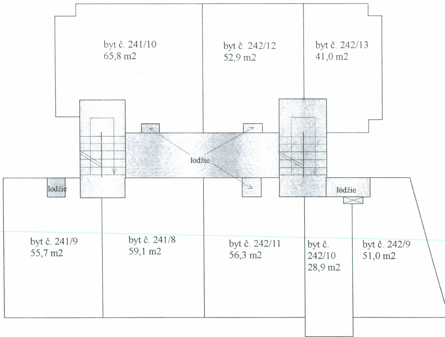
3. nadzemní podlaží
