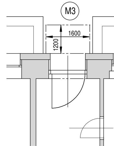
M3 SKLENĚNÁ MARKÝZA O ROZMĚRU 1600x1200mm (délka x vyložení)
