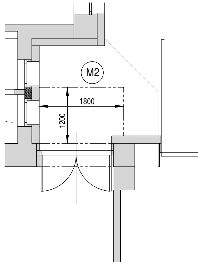
M2 SKLENĚNÁ MARKÝZA O ROZMĚRU 1800x1200mm (délka x vyložení)
