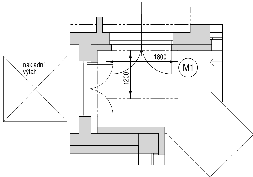
M1 SKLENĚNÁ MARKÝZA O ROZMĚRU 1800x1200mm (délka x vyložení)
