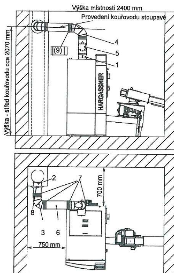
Sada připojovacího potrubí: RLA Ø 150 mm s regulátorem komínového tahu (výr. č.: 7115020)
