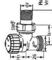
Rohový Vnější závit G 3/4"
