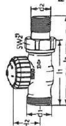
Přímý Vnější závit G 3/4"
