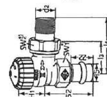
Rohový Viega-SC 15 mm
