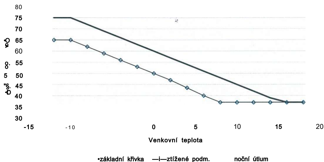
Teplotní diagram
