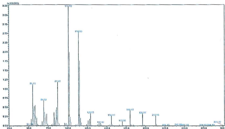
Hmotnostní spektrum látky v retenčním čase 9,7 min: „2-octyl-2H-izothiazol-3-one; CAS č. 26530-20-1“
