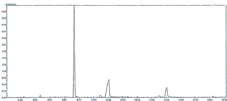
Chromatogram vzorku rohože: pík látky v retenčním čase 9,7 min odpovídá „2-octyl-2H-izothiazol-3-one; CAS č. 26530-20-1“
