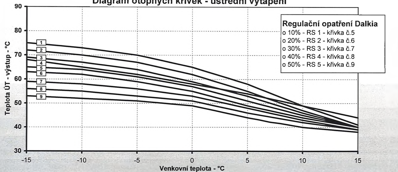
Diagram otopných křivek - ústřední vytápění
