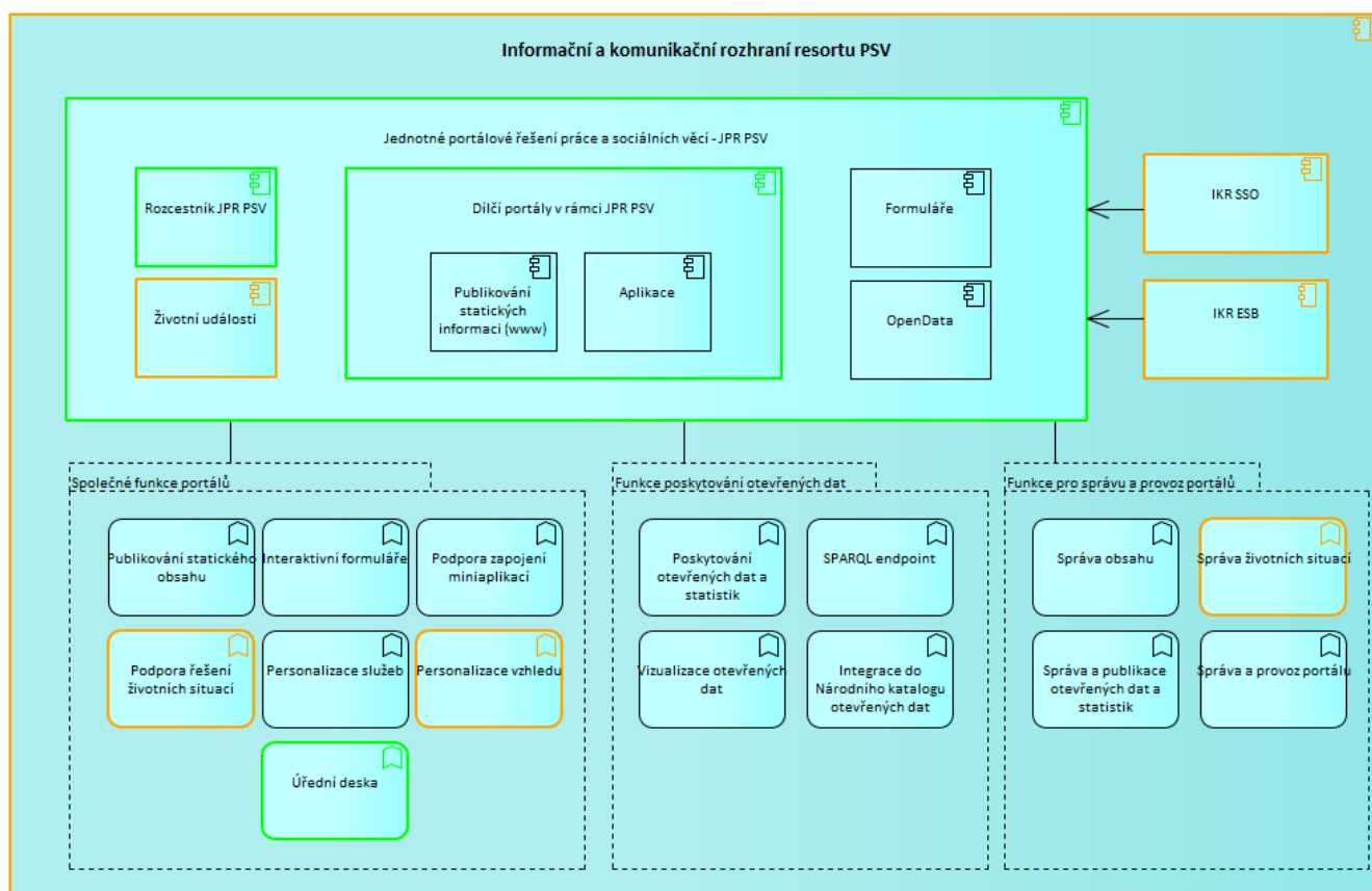
Obrázek 3 Aplikační architektura JPR PSV
