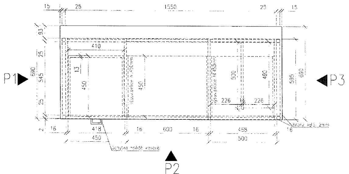
Víceúčelový stůl 1:10
