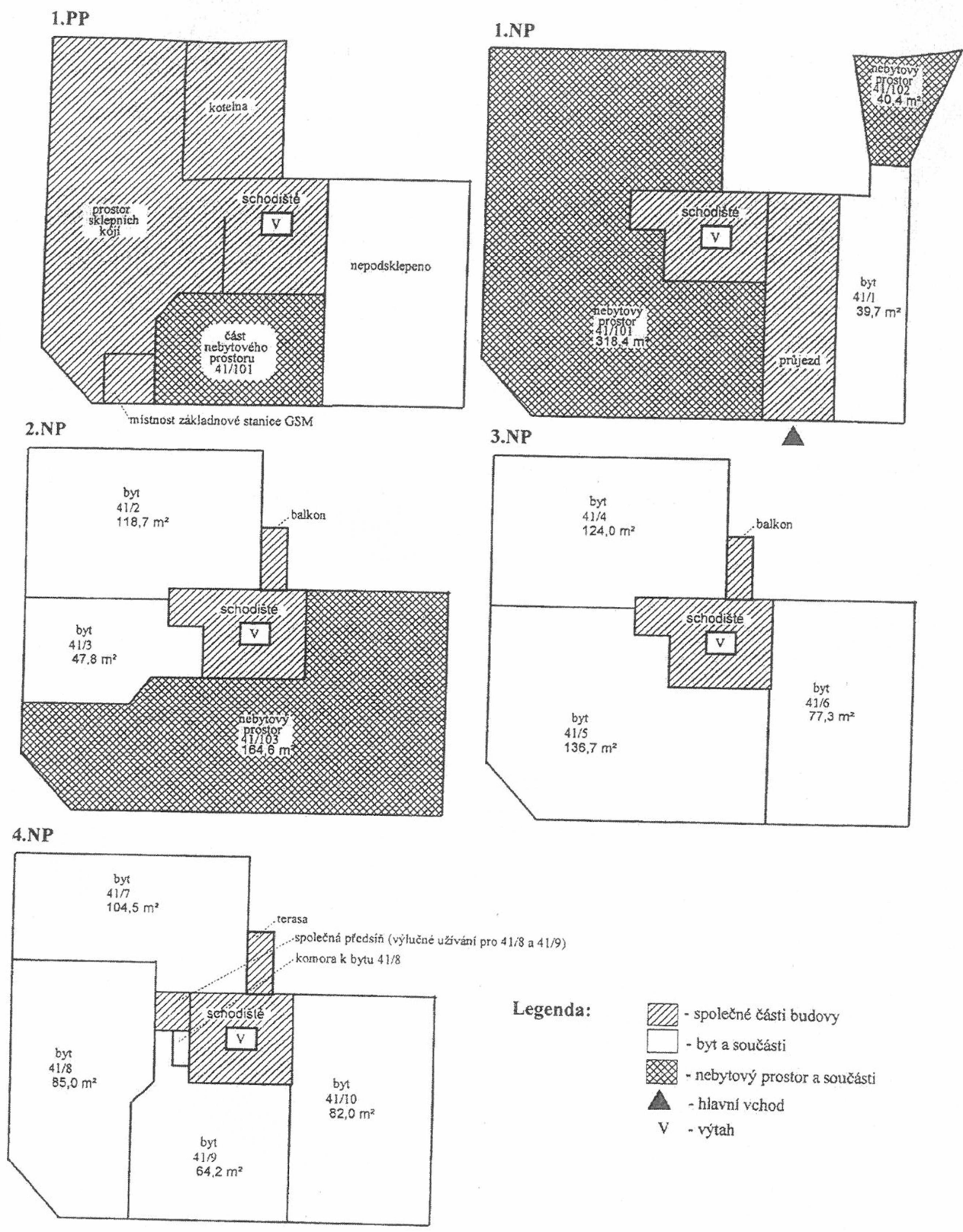
Schema budovy: Rubešova č.p. 41, obec Praha, část obce Vinohrady
