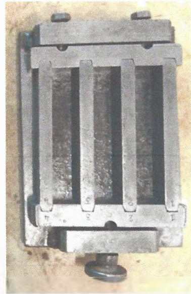
Reálný obrázek ocelové formy 20 x 20 x 100 mm
