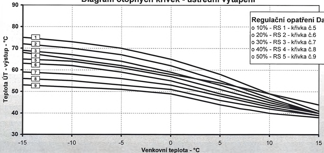
Diagram otopných křivek - ústřední vytápění
