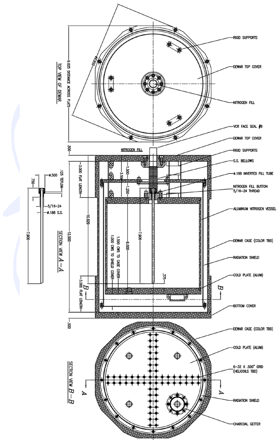
Obrázek č. 1 – Schéma vakuové komory
